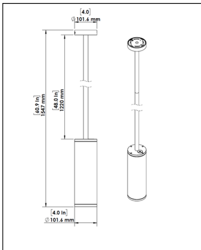
CYLUX4- PENDANT MOUNT
